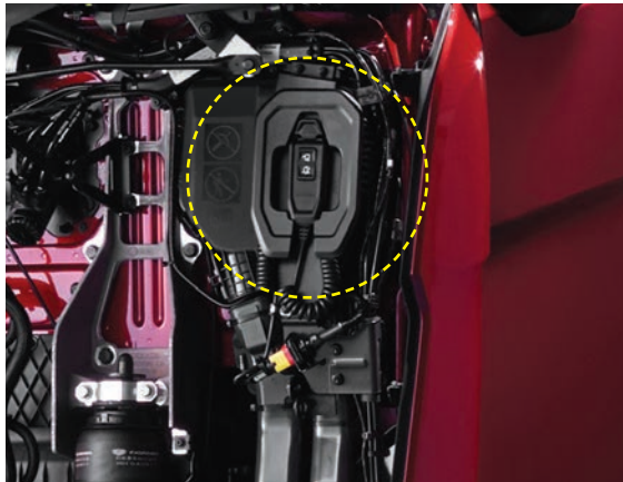
전동 캡틸팅 스위치 프론트 그릴에 위치한 전동 캡틸팅 스위치로 보다 편리하게 캡틸팅 조정이 가능합니다.
