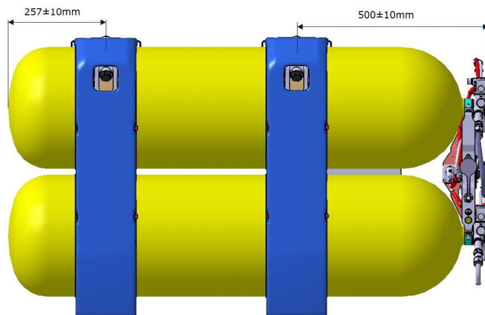
Figura 6: Posicionamento das cintas para cilindros de 80L
