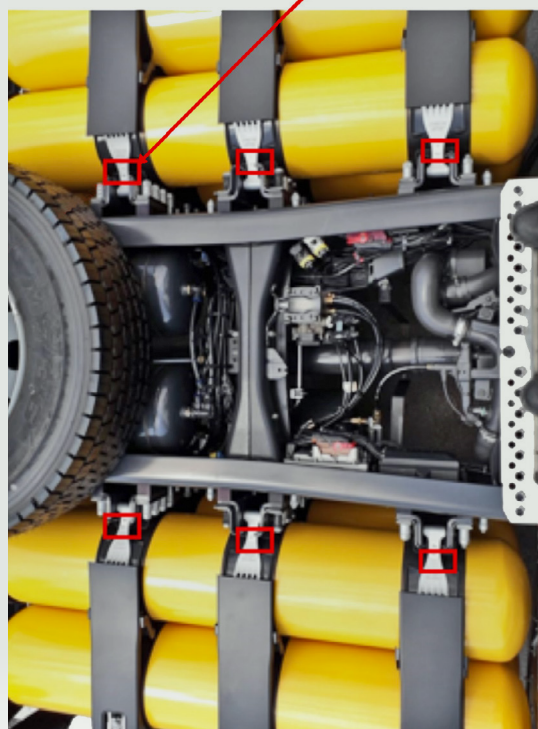
Figura 21: Vista superior, posição das marcações de certificação dos suportes
