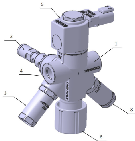
Figura 9.1: Válvula do cilindro com dispositivo de alívio por temperatura por bulbo de vidro
