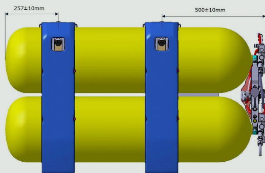
Figura 22: Posicionamento das cintas para cilindros de 80L
