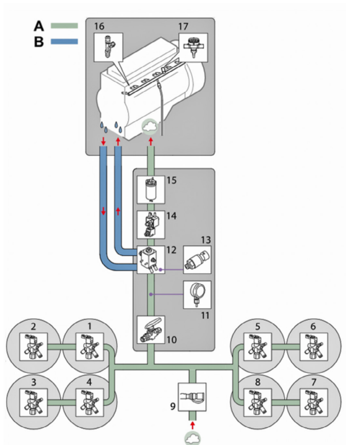
Figura 1: Visão geral do sistema GNV
