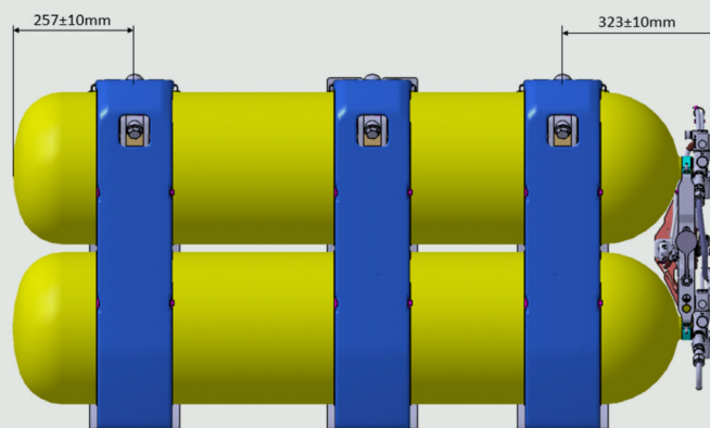
Figura 23: Posicionamento das cintas para cilindros de 95L
