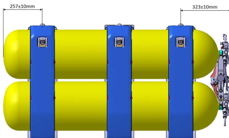
Figura 4: Posicionamento das cintas para cilindros de 95L
