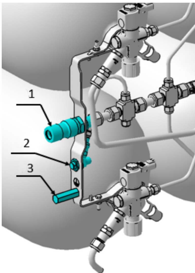
Figura 12: Localização das válvulas de abastecimento
