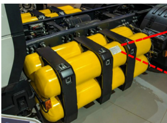
Figura 3.1: Etiqueta de aviso de uso e cuidados na utilização de GNV
