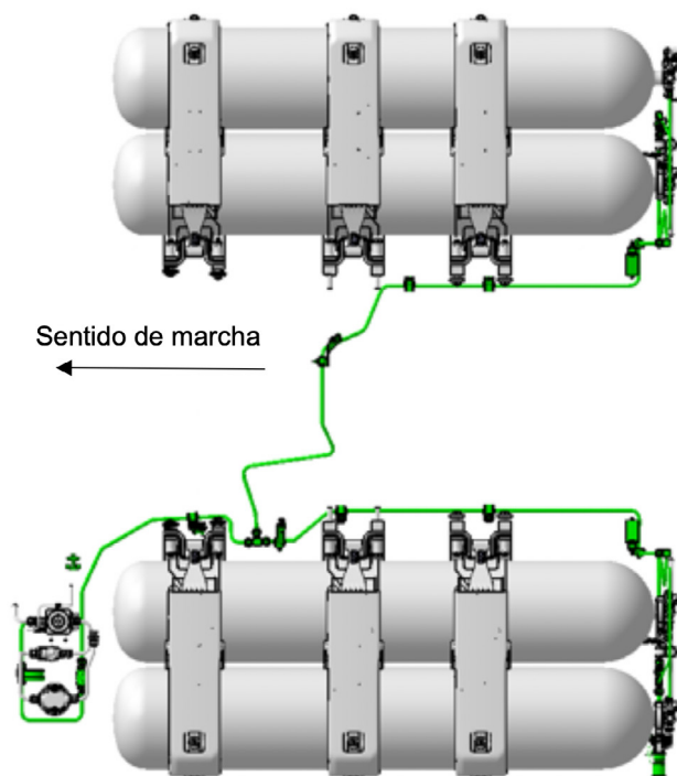
Figura 7: Arquitetura da tubulação de alta pressão na versão somente tubos metálicos
