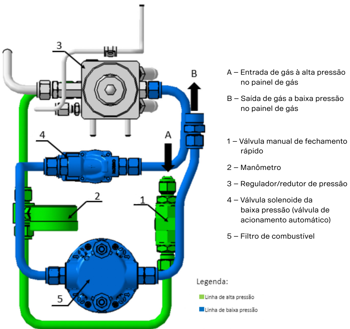
Figura 13: Arquitetura do painel de gás
