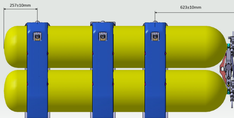
Figura 24: Posicionamento das cintas para cilindros de 118L
