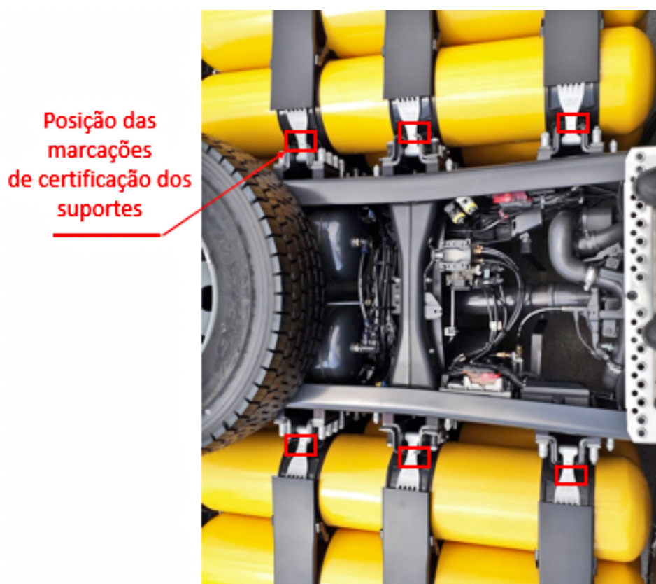
Figura 2: Vista superior, posição das marcações de certificação dos suportes
