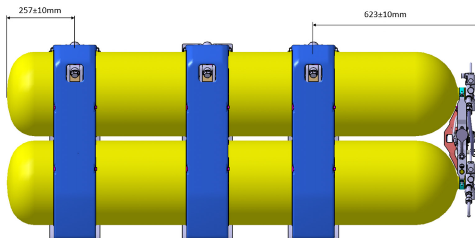
Figura 5: Posicionamento das cintas para cilindros de 118L
