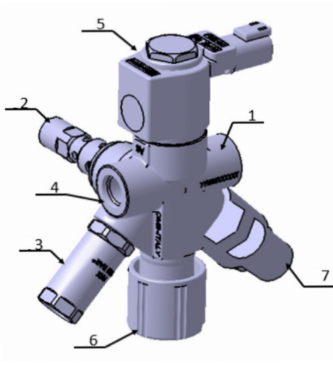
Figura 9: Válvula do cilindro com dispositivo de alívio por temperatura por liga fundível
