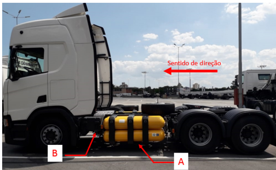
Figura 18: Vista do lado esquerdo do veículo 6x2
