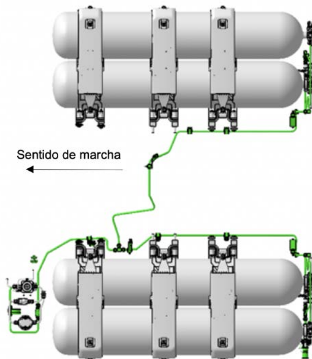
Figura 8: Arquitetura da tubulação de alta pressão na versão somente tubos metálicos
