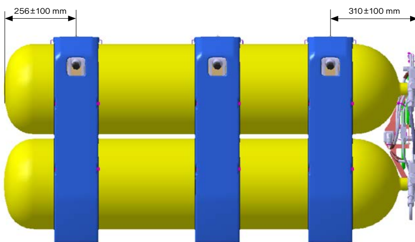
Figura 5: Posicionamento das cintas para cilindros de 95 litros
