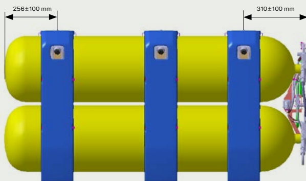
Figura 28: Posicionamento das cintas para o conjunto de cilindros de 95 litros
