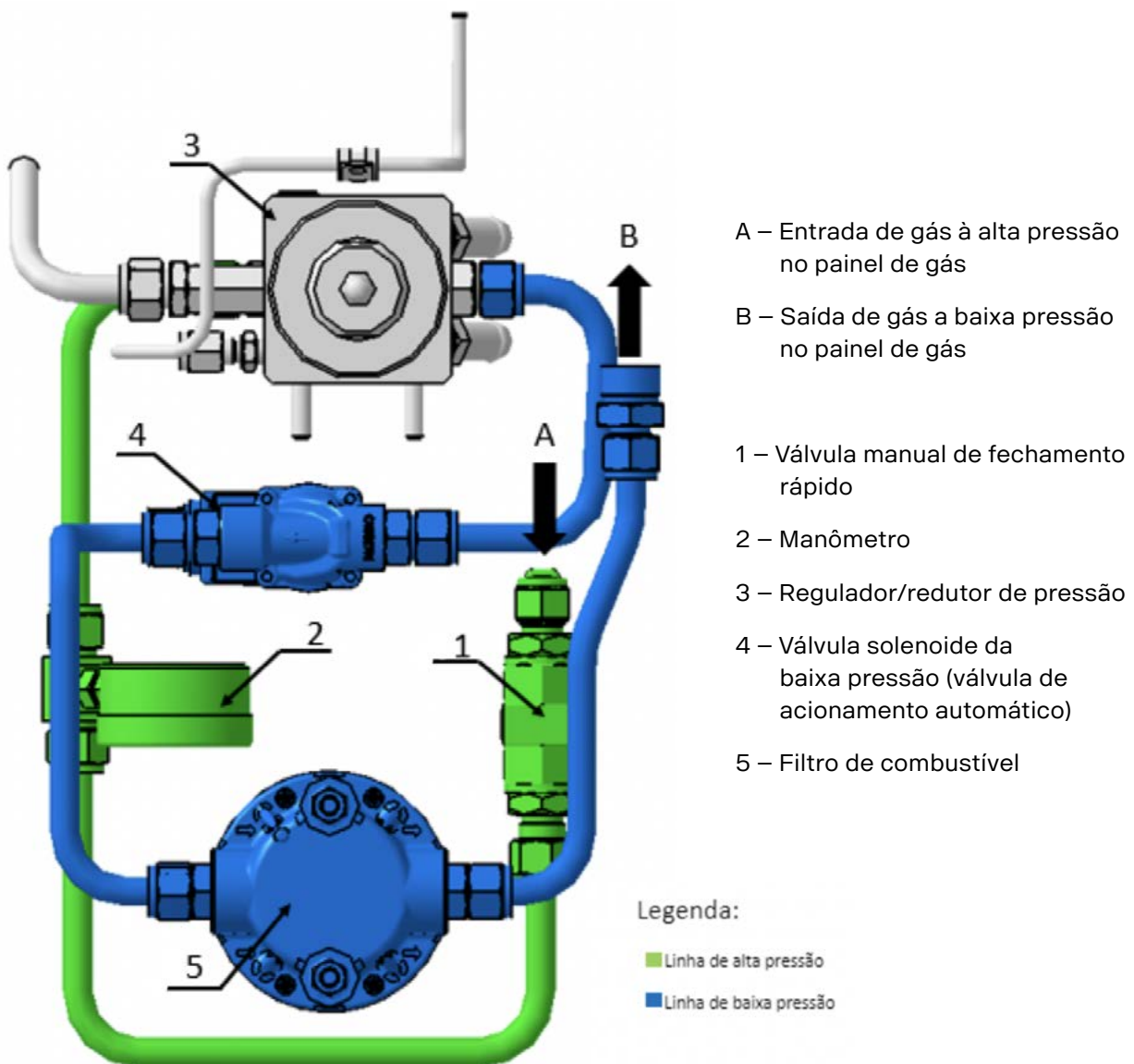
Figura 14: Arquitetura do painel de gás
