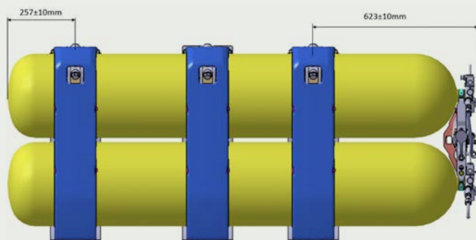
Figura 29: Posicionamento das cintas para o conjunto de cilindros de 118 litros
