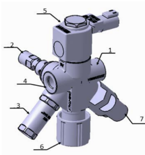
Figura 10: Válvula do cilindro com dispositivo de alívio por temperatura por liga fundível
