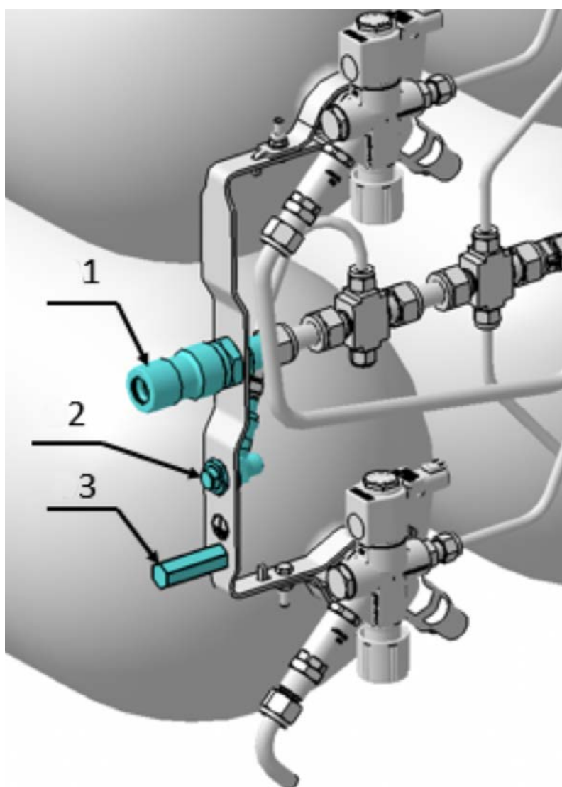
Figura 13: Localização das válvulas de abastecimento
