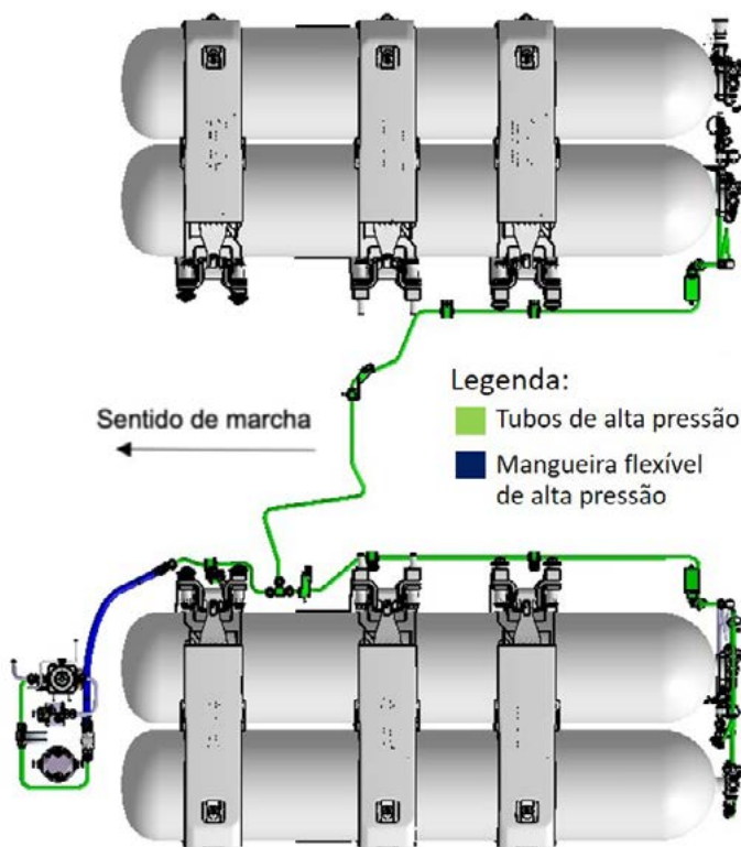
Figura 8.1: Arquitetura da tubulação de alta pressão na versão que contém mangueira flexível.
