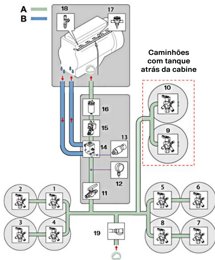
Figura 1: Visão geral do sistema GNV
