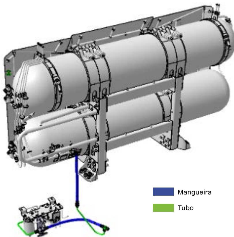
A figura 8.2: mostra a tubulação de alta pressão na versão que contém tubos metálicos e mangueiras flexíveis.
