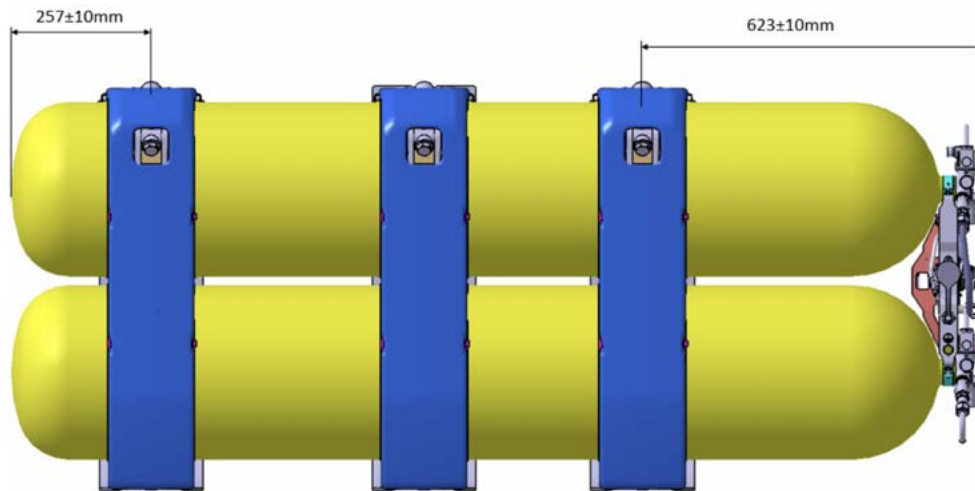
Figura 6: Posicionamento das cintas para cilindros de 118 litros
