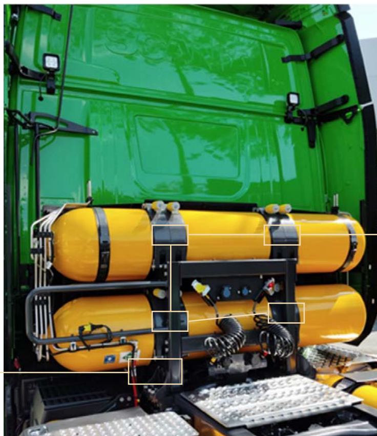
Figura 3: Vista traseira das marcações de certificação dos suportes e cintas
