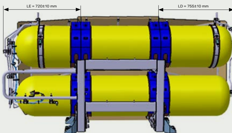
Figura 30: Posicionamento das cintas para o conjunto de cilindros de 235 litros atrás da cabine
