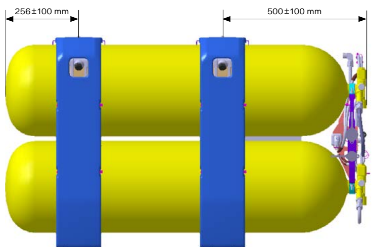
Figura 4: Posicionamento das cintas para cilindros de 80 litros
