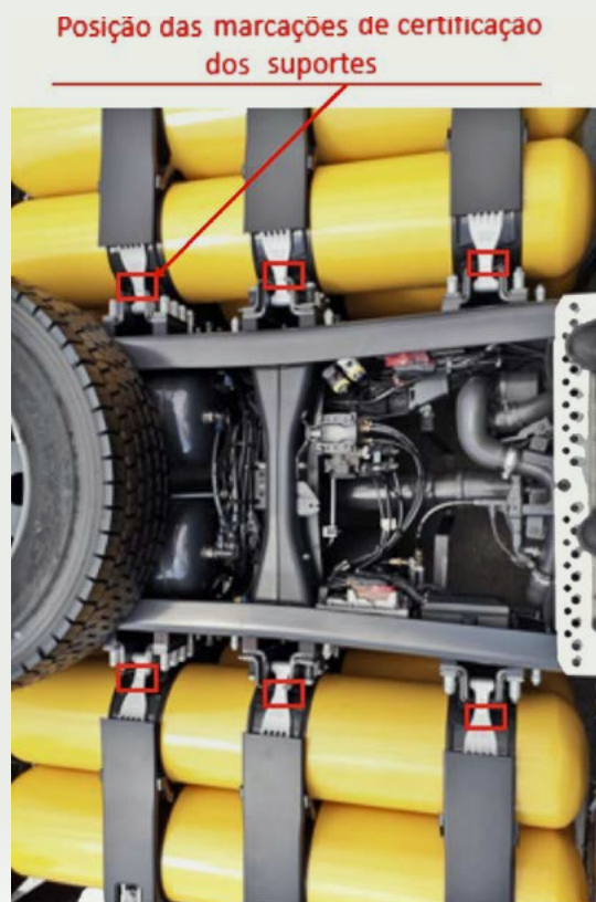
Figura 25: Vista superior, posição das marcações de certificação dos suportes
