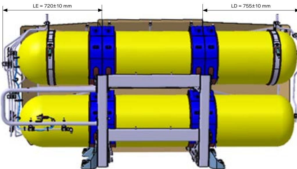
Figura 7: Posicionamento das cintas para cilindros de 235 litros
