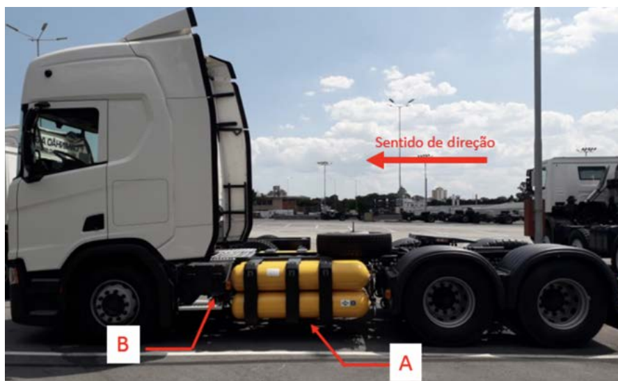
Figura 21: Vista do lado esquerdo do veículo 6x2
