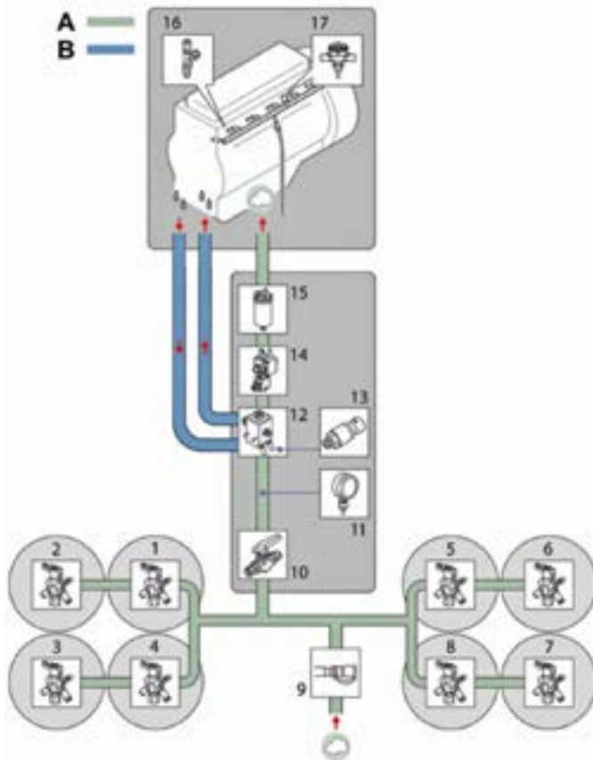
Figura 1: Visão geral do sistema GNV
