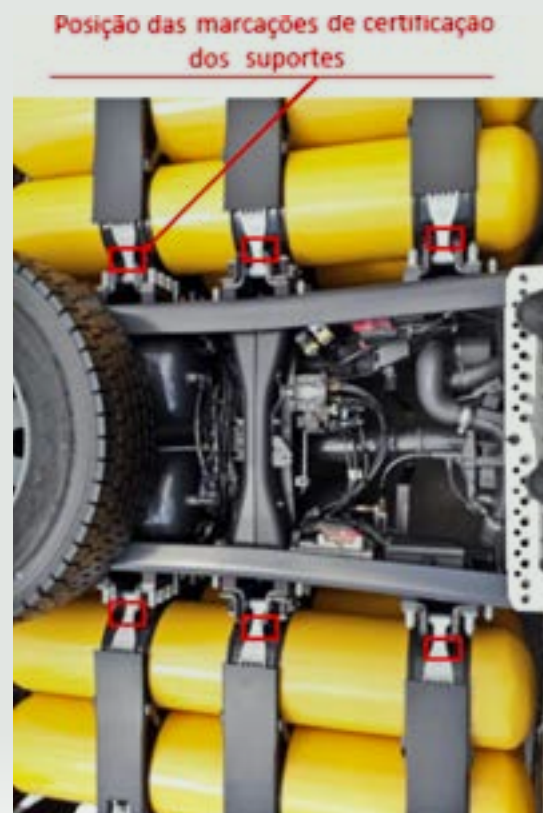
Figura 21: Vista superior, posição das marcações de certificação dos suportes
