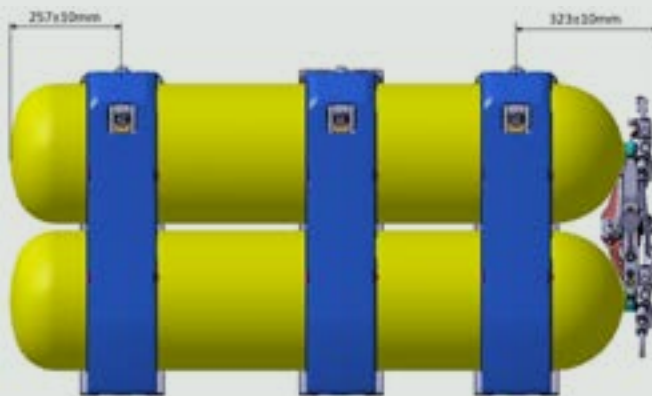
Figura 23: Posicionamento das cintas para cilindros de 95L
