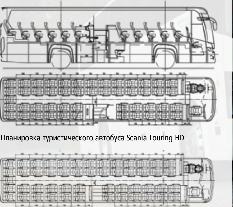
Планировка междугородного автобуса Scania Touring HD
