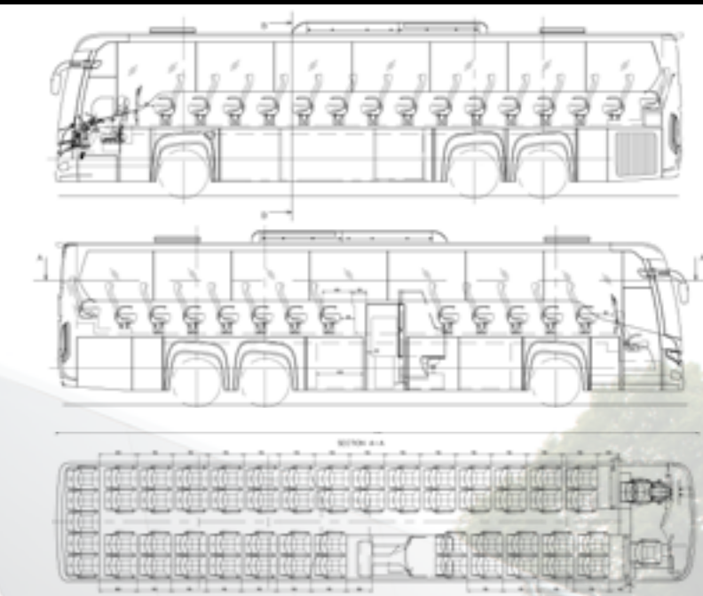
Планировка туристического автобуса Scania Touring HD
