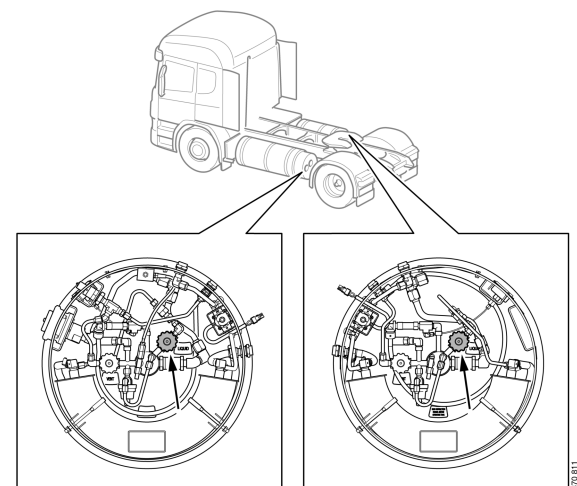
断流旋塞
