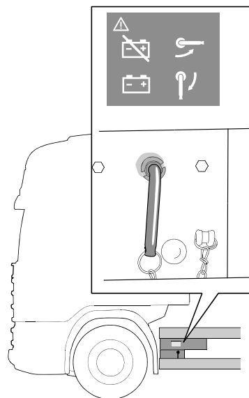
蓄电池总开关把手
