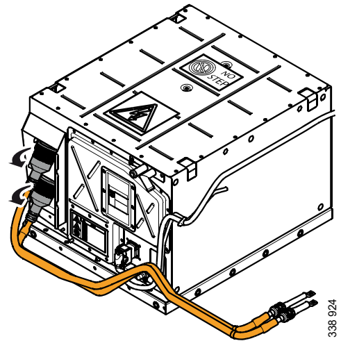
断开油电混合车蓄电池上的接头。
