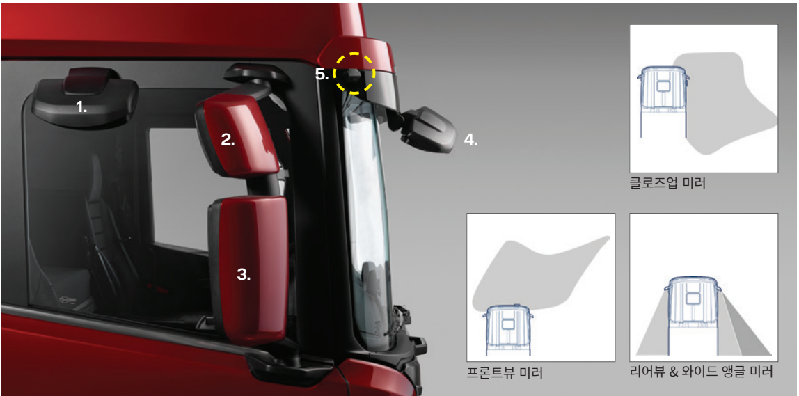
1. 클로즈업 미러 2. 와이드 앵글 미러 3. 리어뷰 미러 4. 프론트뷰 미러 5. 전방 사각지대 카메라
